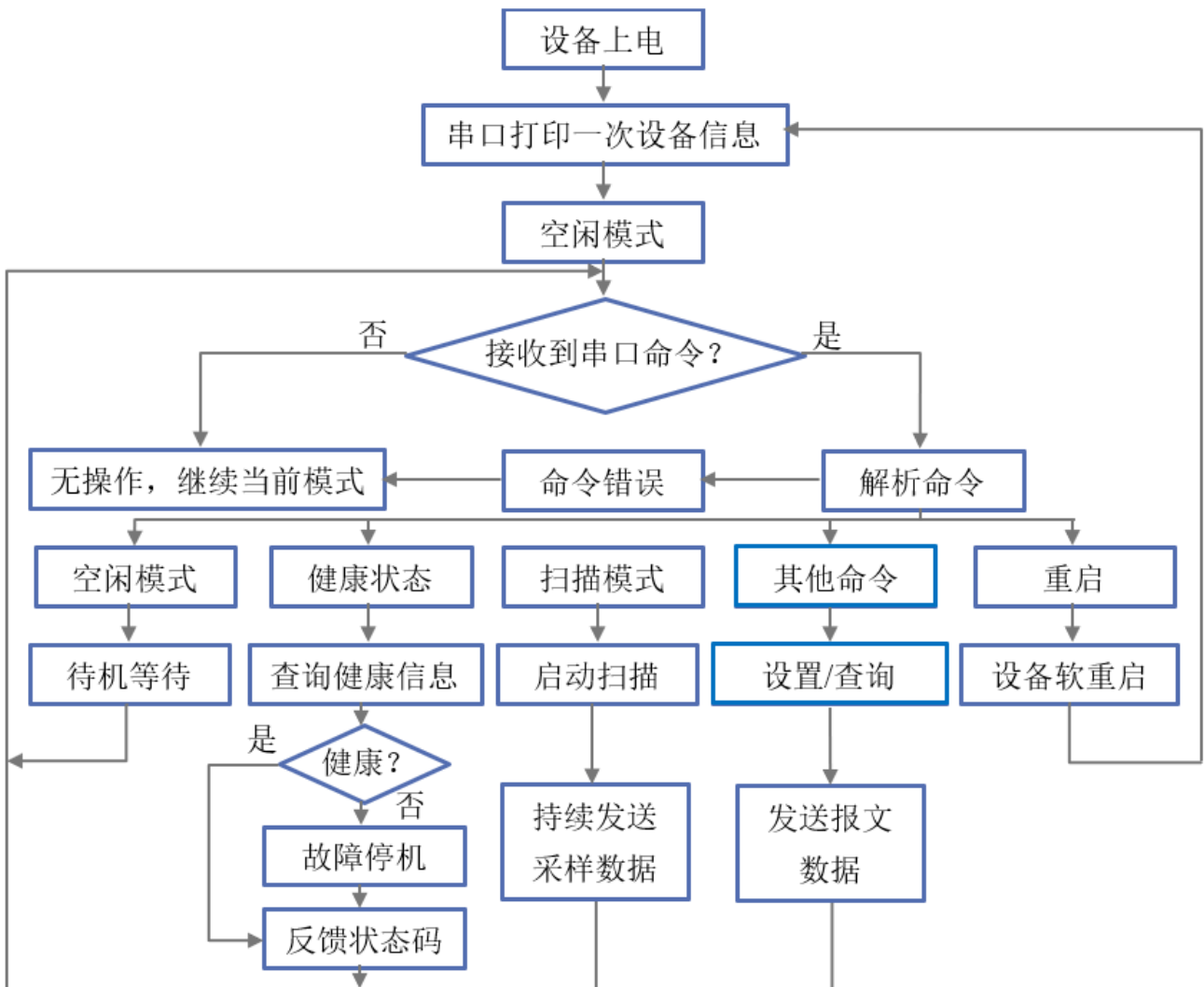
图 1 YDLIDAR G4 系统工作流程图
