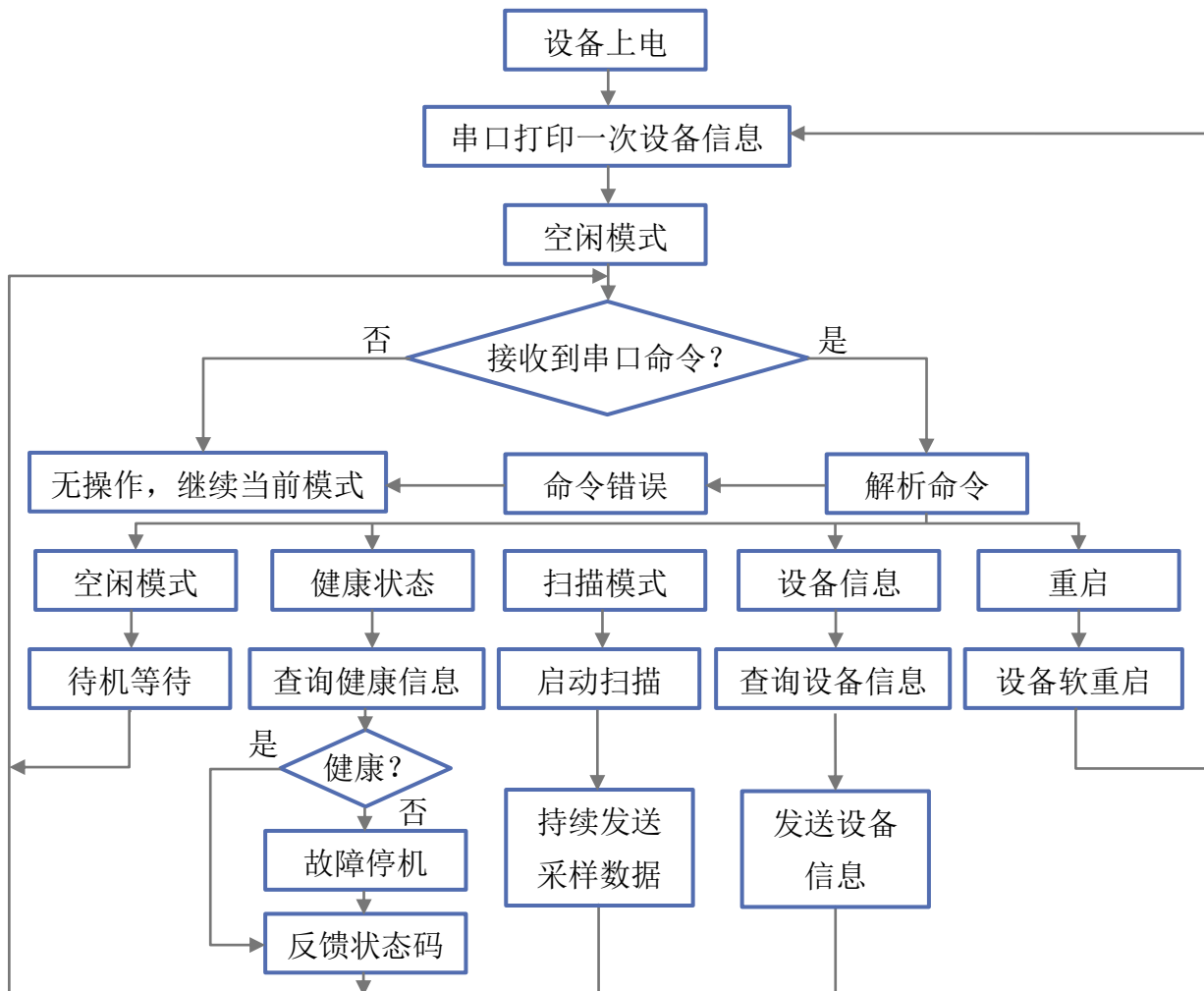
图 1 YDLIDAR X4 系统工作流程图
